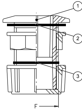
Kit bocchettone di scarico completo di guarnizioni. Bianco - atossico Tank outlet kit with gaskets. White - non-toxic Kit goulotte de vidange avec joint. Blanc - non toxique
